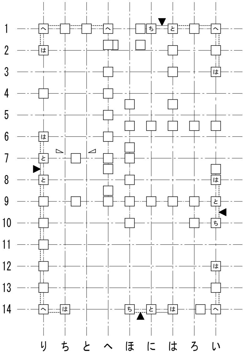
1 階柱壁伏図
