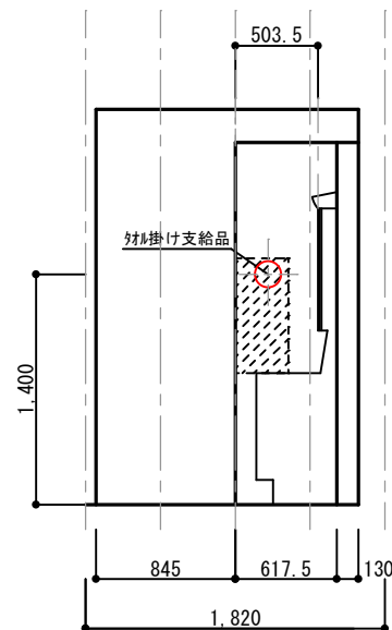
洗面 西面
