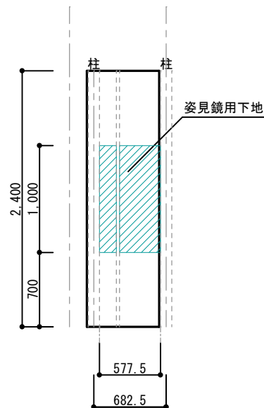
SC 西面
